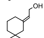
E grandlure II
