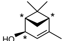
trans -verbenol
