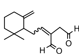
ancistrodial
