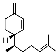
\beta -sesquiphellandrenel
