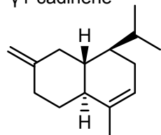
\gamma 1-cadinene
