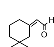
grandlure VI
