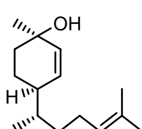
zingiberenol
