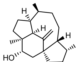
longipenol
