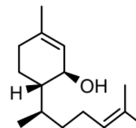
sesquiperitol
