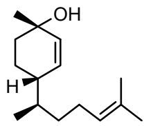
zingiberenol
