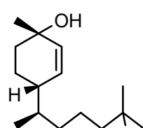
murgantiol
