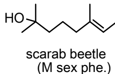
E-subaeneol
