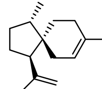
\alpha -acoradiene
