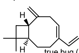
leptotriene
