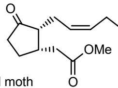
methyl epijasmonate
