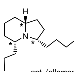
ant (allomone ?)
