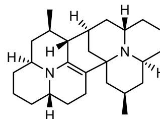
isopsylloborine A
