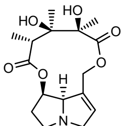
monocrotaline
