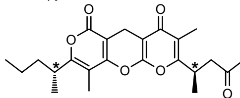
catalipyrone I
